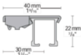
Support à clic pour plafond
