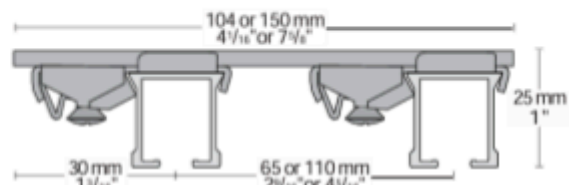
Support à clic pour plafond Double
