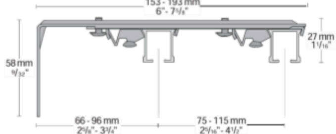
Support mural réglable double
